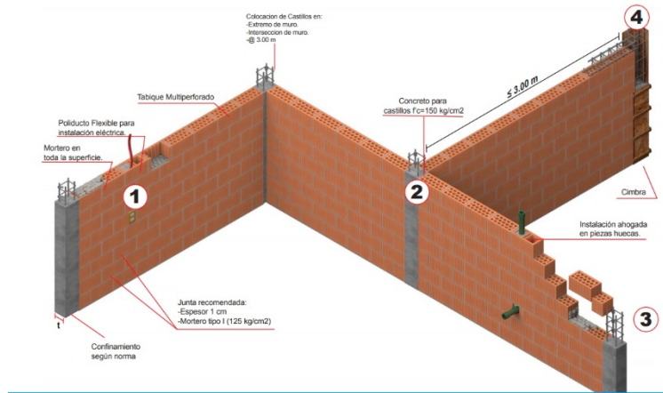
Figura 17: Distribución de mochetas
