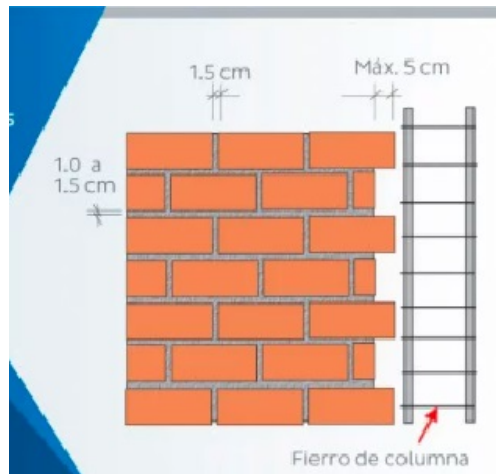
Figura 15: Espesor del mortero entre ladrillos
