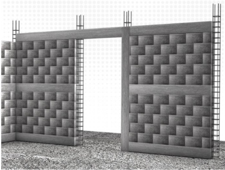
Figura 16: Mocheta en mampostería reforzada
