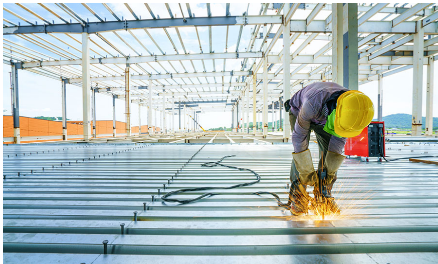
Figura 11: instalación del losacero PSI Concreto
